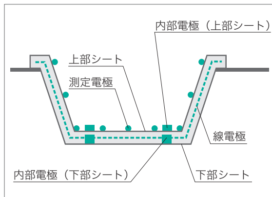
漏水検知システムイメージ図
